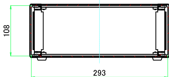
B-B ( 1 : 5 )
